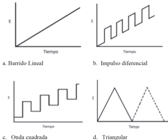
Fig. 1 Señales de excitación en voltamperometría cíclica.
