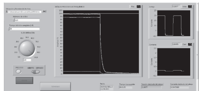
Fig. 8. Señal onda cuadrada.
