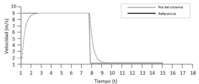
Fig. 11. Respuesta de velocidad de la banda transportadora.
