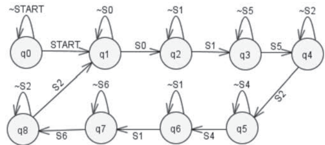
Fig. 2. Diagrama de estados del proceso.
