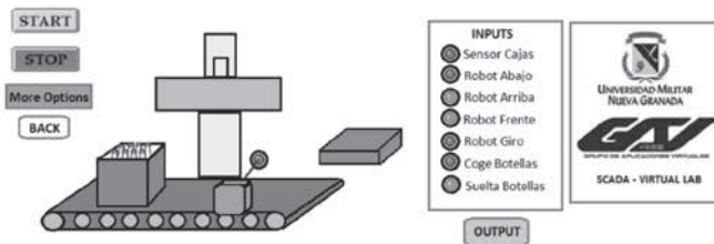
Fig. 9. SCADA del Laboratorio virtual desarrollado.
